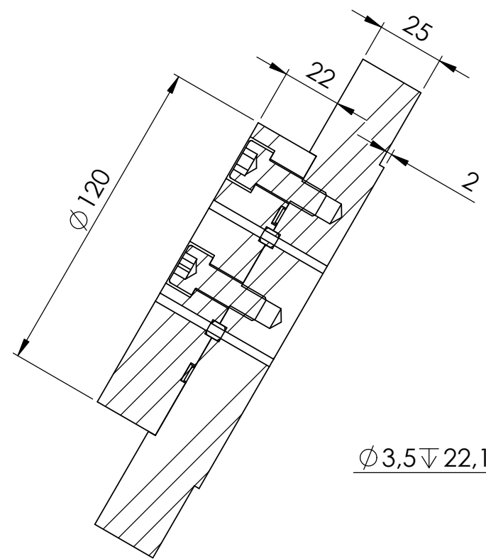
SCHNITT A-A
