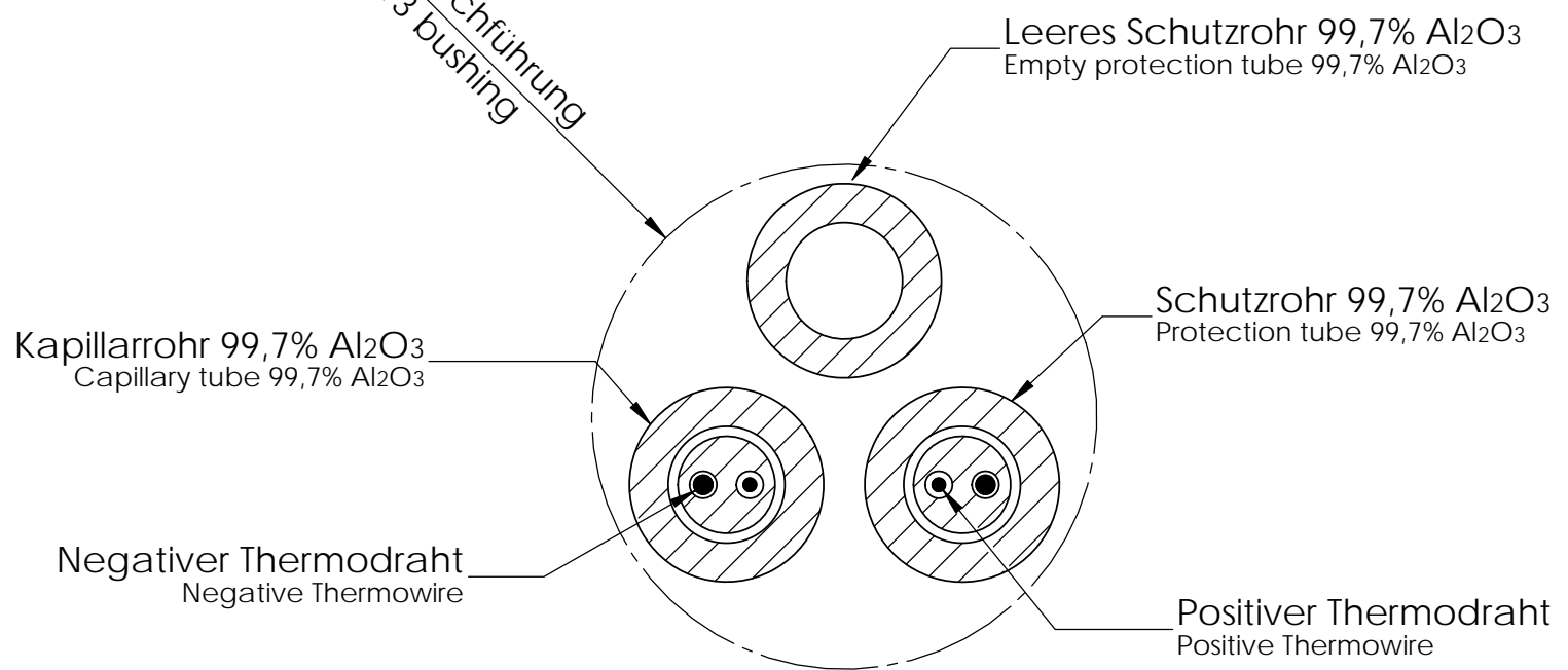
SCHNITT A-A MAßSTAB 5 : 1
